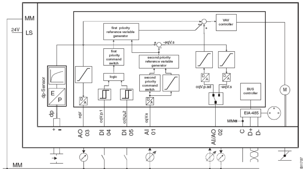
Схема подключения
